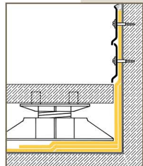
Perfil reversível e empilhável
