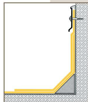
Perfil de parede simples
